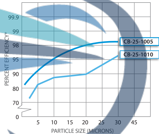
2.5" Diametro x 9 7/8" Largo
